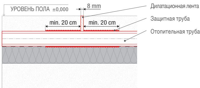
Рисунок 8: Защита FV PE отопительных труб во время перехода через дилатационный шов защитной трубой.
