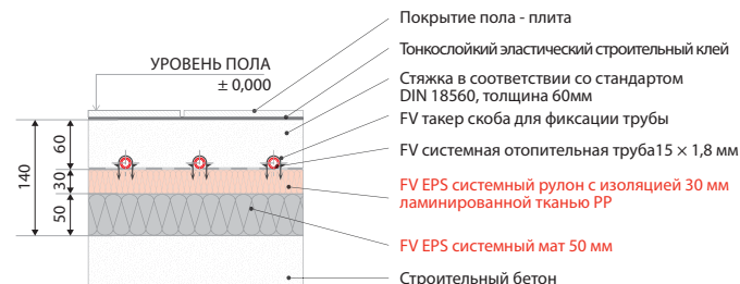
Рисунок 18: Рекомендуемый состав пола над открытым пространством в соответствии со стандартом ČSN EN 1264 термостойкость изоляции R=2,00 м² K/W
