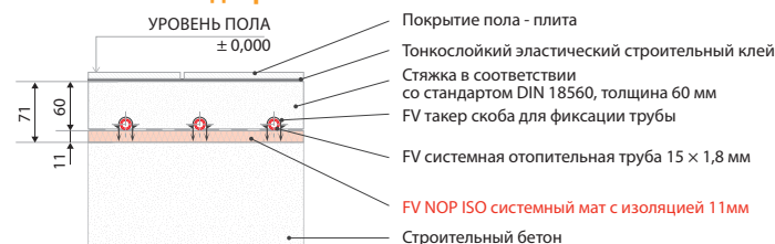
Рисунок 16: Рекомендуемый состав пола над отопляемыми помещениями в соответствии со стандартом ČSN EN 1264 термостойкость изоляции R=0,75 м² K/W
